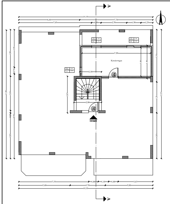
Σχήμα 3: Κάτοψη ισογείου
