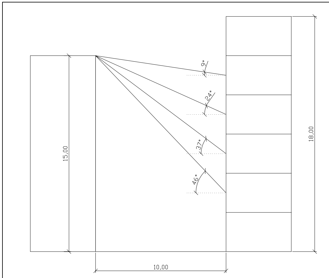
Σχήμα 7: Γωνίες σκίασης νότια όψης από μακρινά εμπόδια
