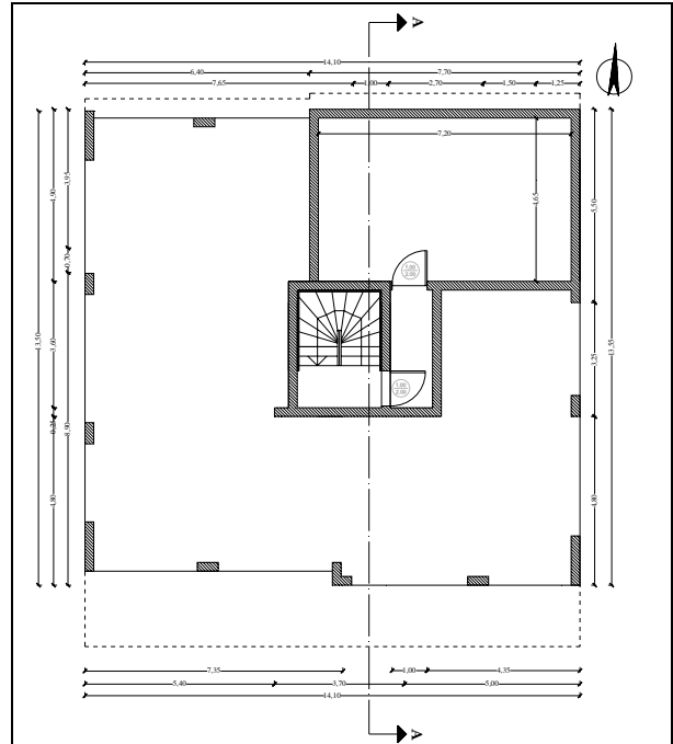
Σχήμα 4: Κάτοψη υπογείου
